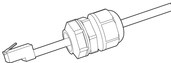
Figura 25 - Montaggio del connettore di comunicazione
