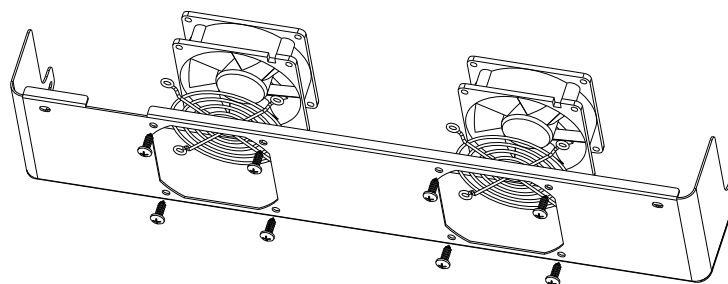
Figura 41 - Rimozione della ventola e del coperchio di protezione
