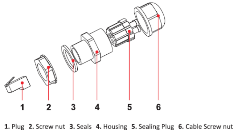
Figura 23 – Connettore per la comunicazione tramite la porta 485
