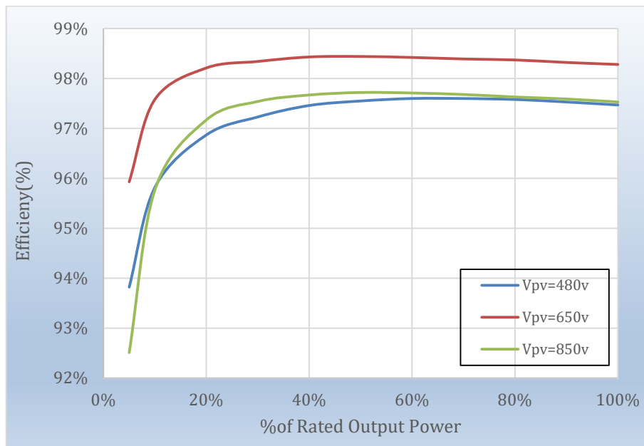
Figura 10 - Curva di efficienza energetica (ad esempio 20 kW)
