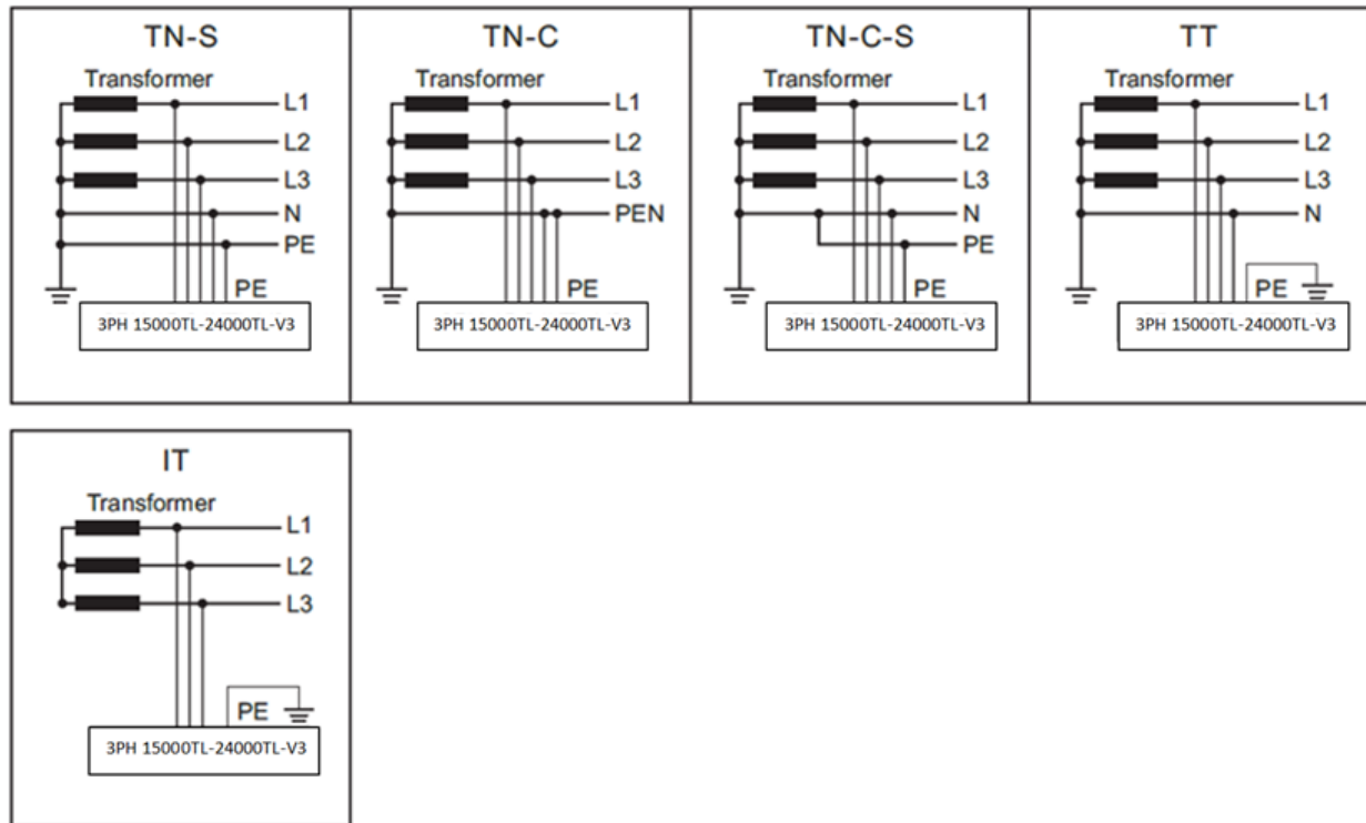
Figura 3 - Schemi elettrici dei tipi di rete su cui è possibile installare l'inverter 3PH 15000TL-24000TL-V3
