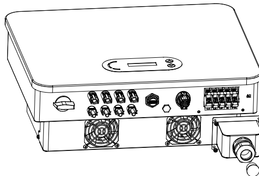
Figura 19 - Collegamento dei cavi di uscita CA (1)
