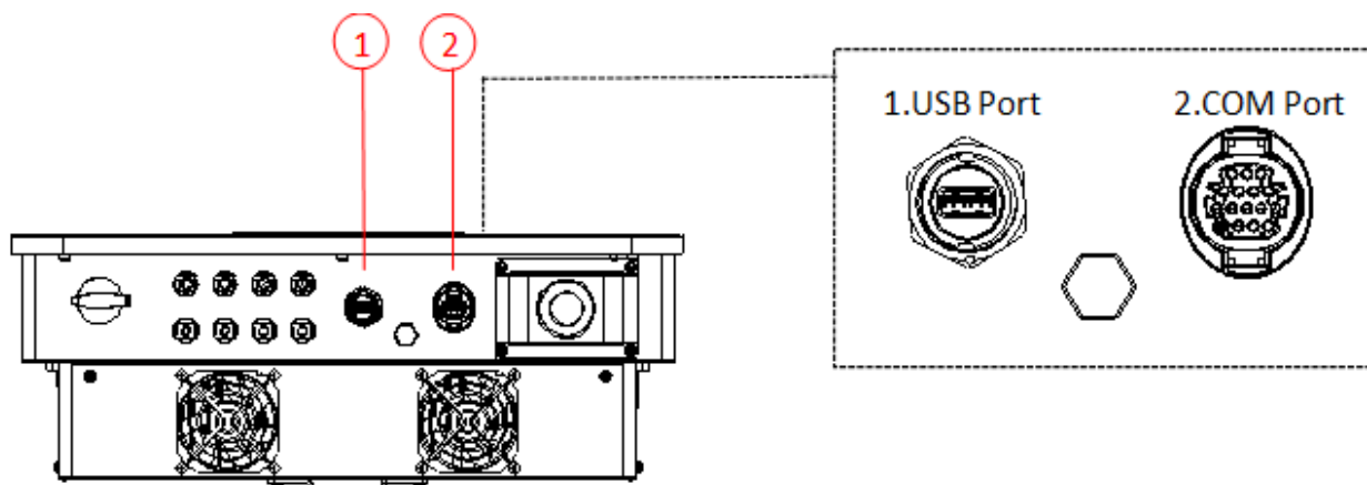
Figura 22 - Vista dal basso dell'inverter 3PH 15000TL-24000TL-V3
