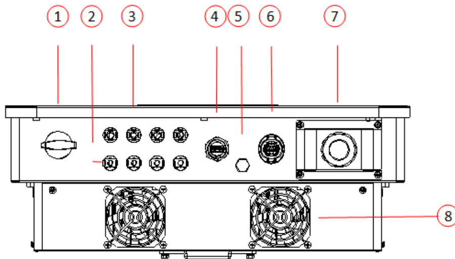
Figura 7 - Vista dal basso dell'inverter
