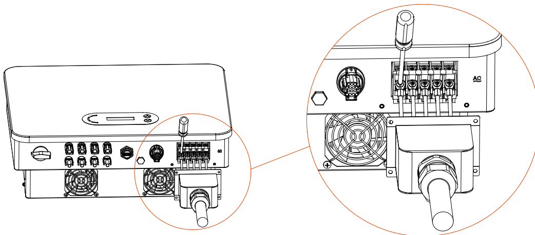
Figura 21 - Collegamento dei cavi di uscita CA (3)
