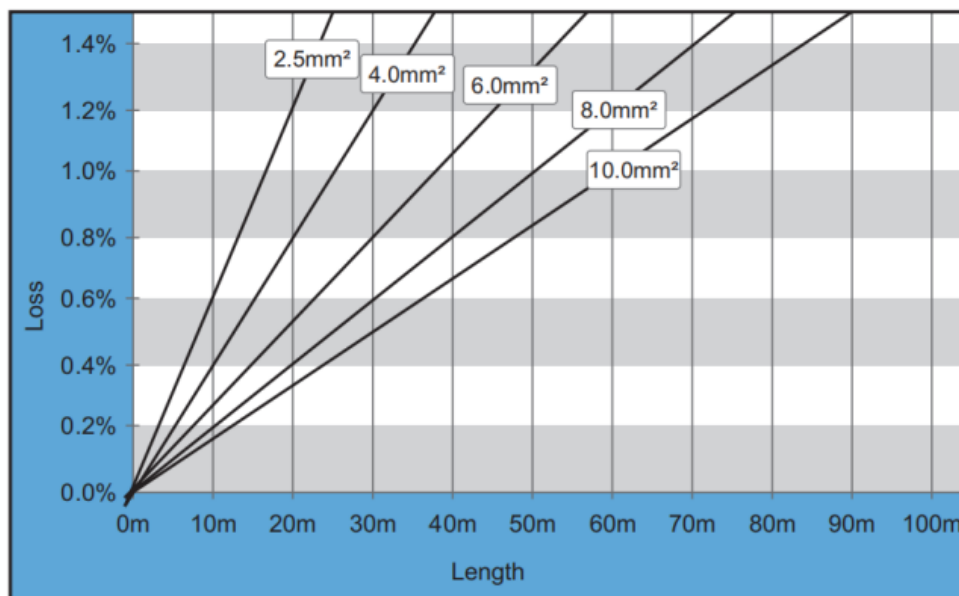
Figura 30 - Relazione tra lunghezza del cavo, area della sezione trasversale e potenza dissipata
