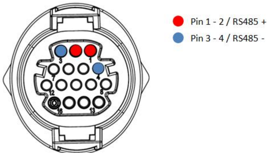
Figura 85 – Collegamento della linea seriale tramite connettore di comunicazione per 3PH HYD5000-HYD20000-ZSS
