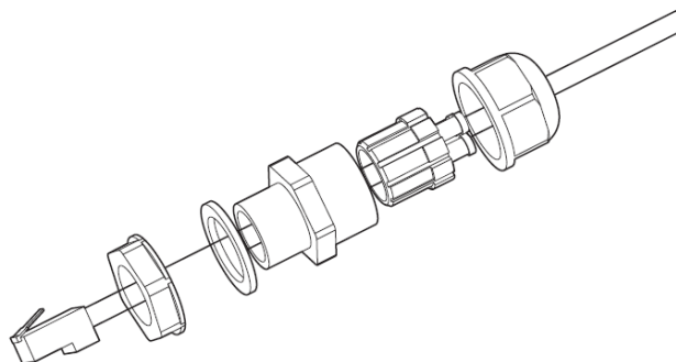
Figura 24 - Montaggio del connettore di comunicazione
