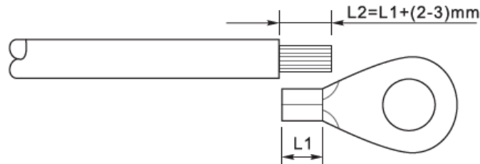
Figura 10 - Preparazione del cavo di terra (1)
