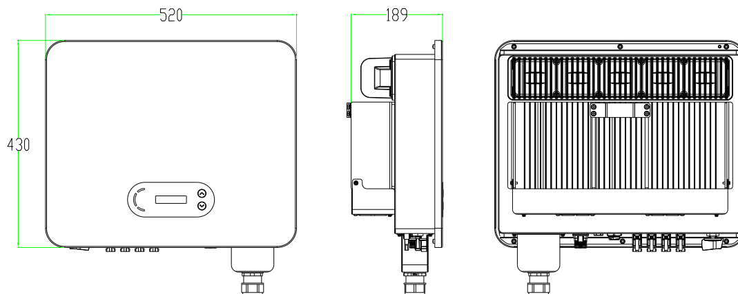
Figura 4 - Vista frontale, laterale e posteriore dell'inverter
