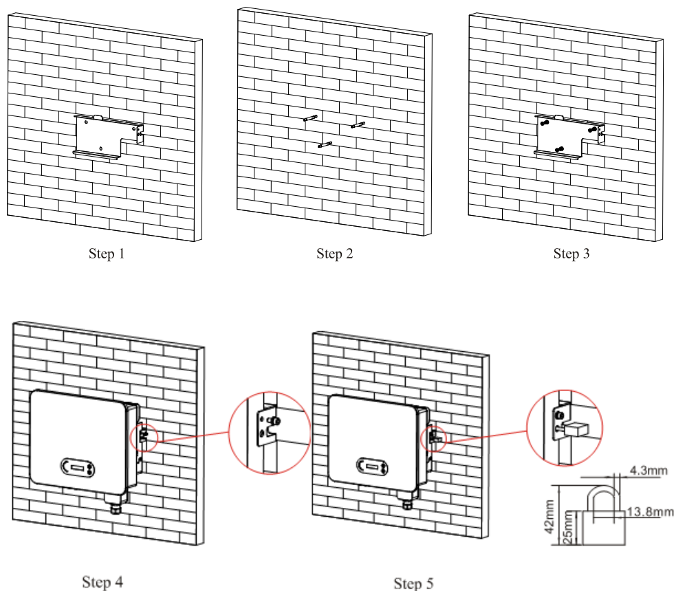
Figura 8 - Fasi per il montaggio dell'inverter a parete
