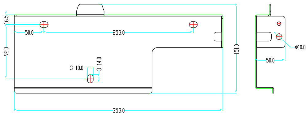
Figura 6 - Dimensioni della staffa
