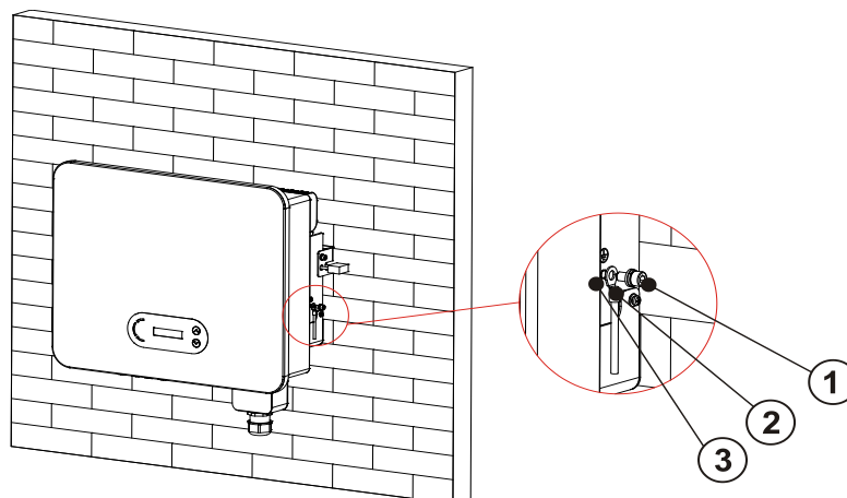
Figura 22 - Schema delle istruzioni di messa a terra esterna dell'inverter
