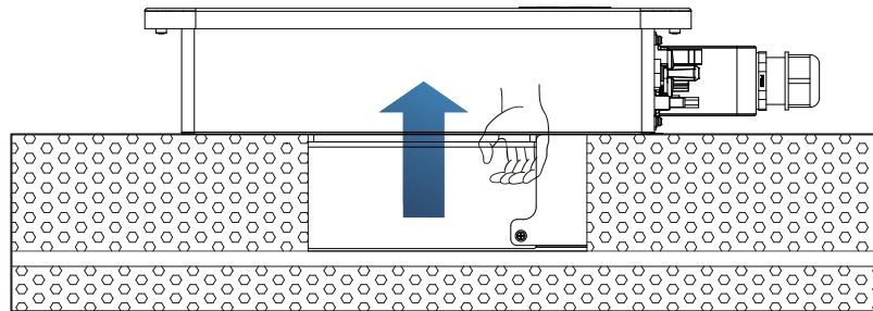
Figura 6 - Rimozione delle protezioni in polistirolo
