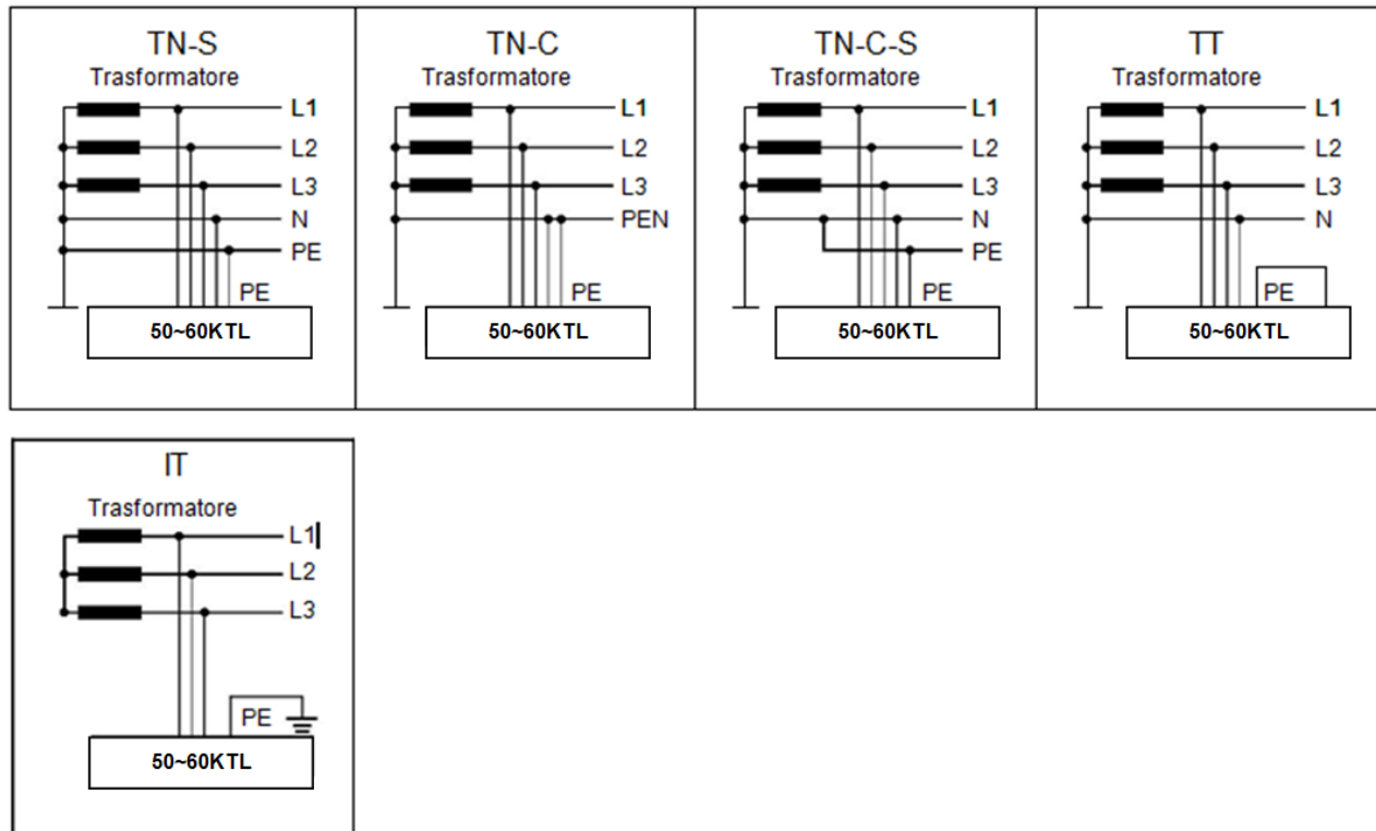
Figura 3 - Schemi elettrici dei tipi di rete su cui poter installare gli inverter 3PH 50000TL-60000TL-V1
