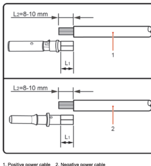
Figura 22 – Connessione dei cavi di potenza DC in ingresso (1)
