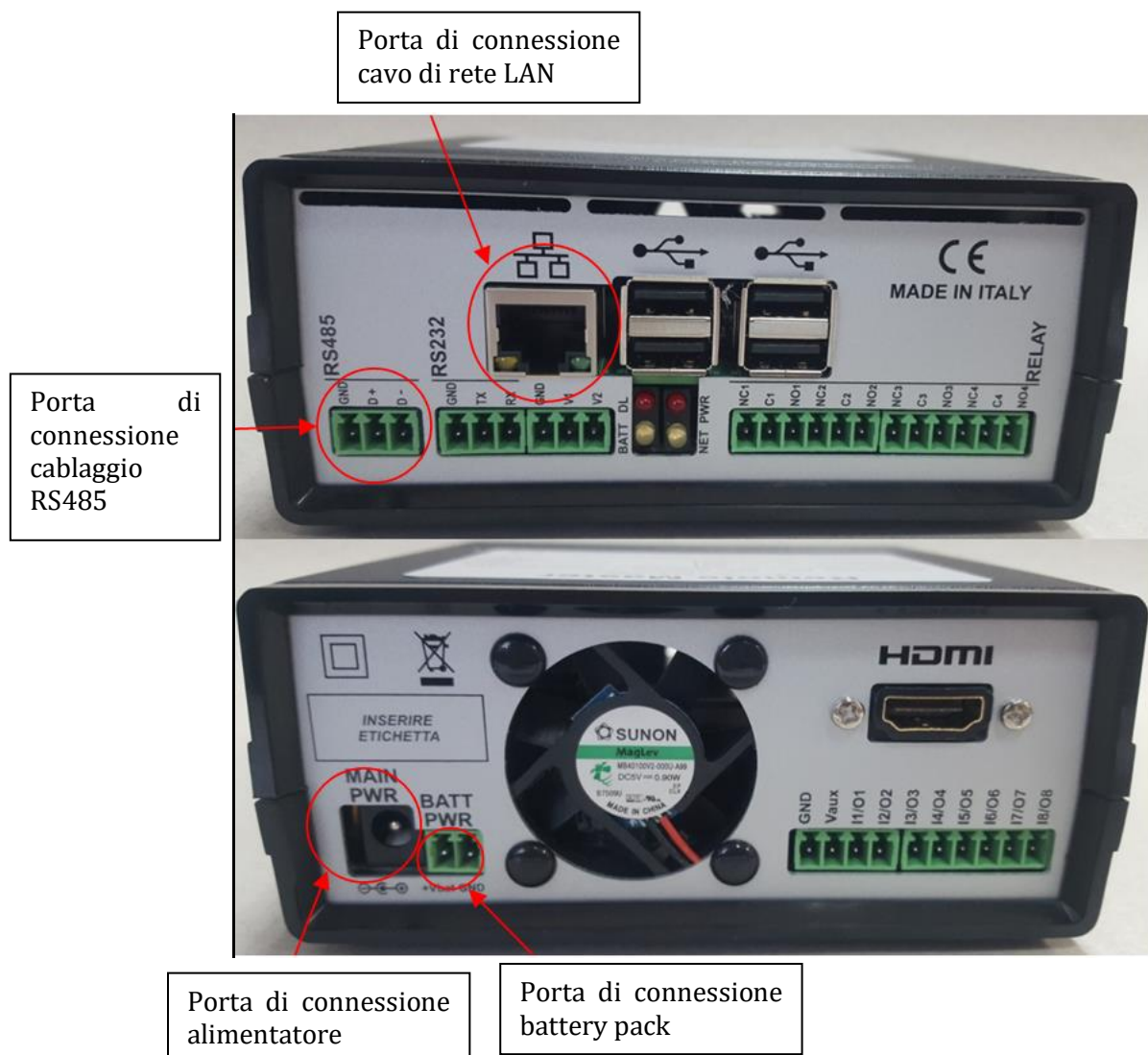
Figura 102: Back Datalogger
