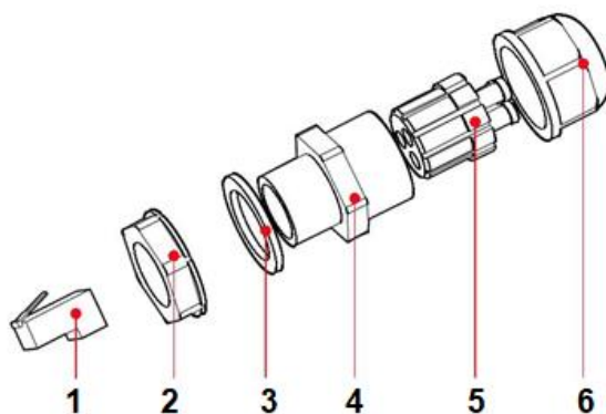
1. Morsetto 2. Ghiera 3. Tenuta 4. Alloggiamento 5. Tappo di tenuta 6. Dado di tenuta
