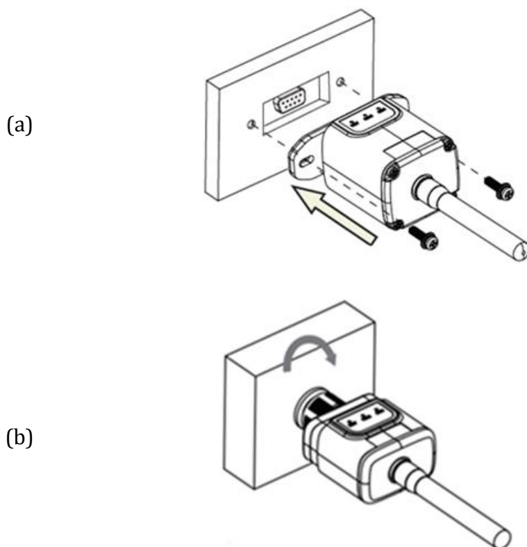
Figura 72 – Inserimento e fissaggio della scheda 4G
