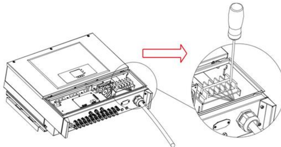
Figura 29 - Connessione dei cavi AC di uscita (3)
