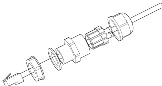
Figura 32 – Montaggio del connettore di comunicazione
