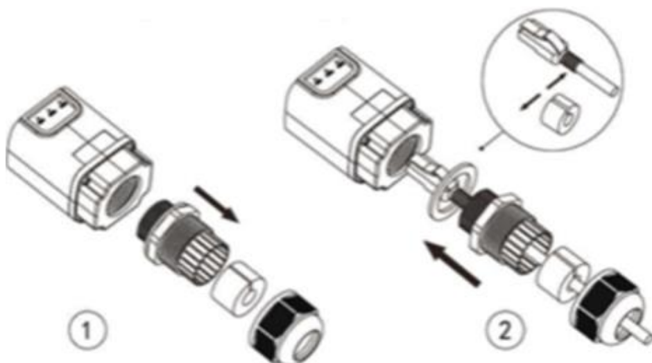
Figura 64 – Inserimento del cavo di rete all'interno del dispositivo
