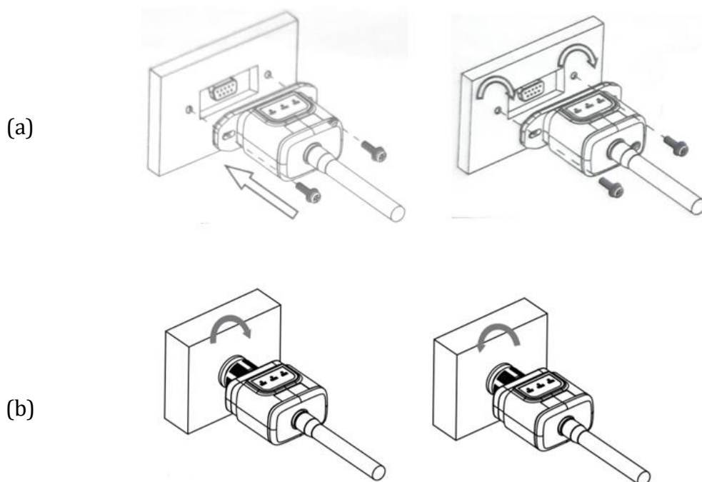
Figura 39 – Inserimento e fissaggio della scheda wifi esterna
