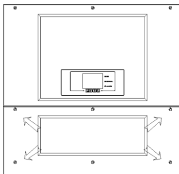
Figura 37 – Estrazione del coperchio centrale
