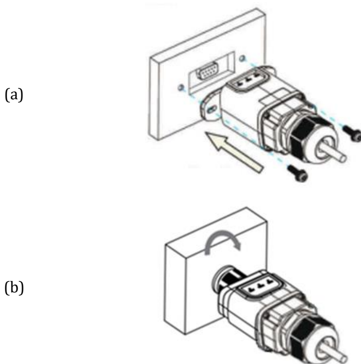
Figura 65 – Inserimento e fissaggio della scheda ethernet
