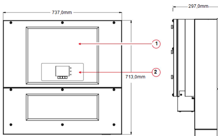
1. Coperchio frontale 2. Interfaccia display
