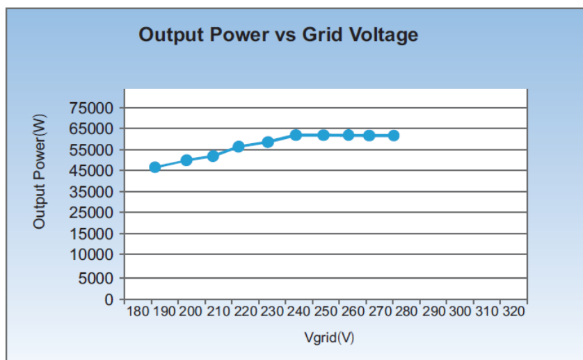
Figura 10 - Curva di derating della tensione in uscita per un inverter Azzurro ZCS della famiglia 3PH 50000TL-60000TL-V1
