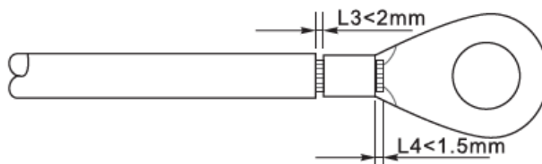
Figura 20 – Preparazione del cavo di terra (2)
