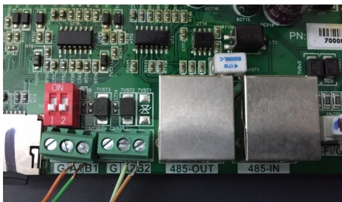
Figura 81 - Collegamento linea seriale tramite morsettiera RS485 e tramite plug RJ45
