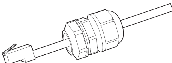
Figura 33 – Montaggio del connettore di comunicazione
