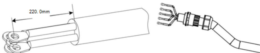
Figura 28 - Connessione dei cavi AC di uscita (2)
