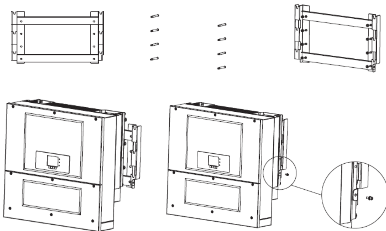
Figura 16 – Passaggi per l'installazione a parete dell'inverter
