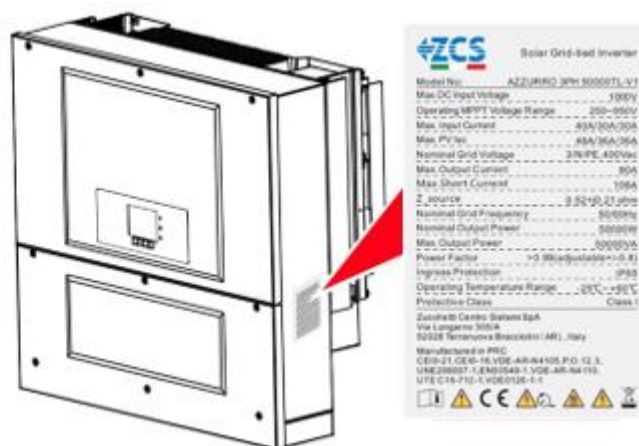
Figura 6 - Non rimuovere l'etichetta posta sul lato dell'inverter
