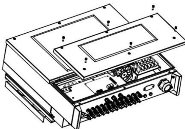
Figura 27- Connessione dei cavi AC di uscita (1)
