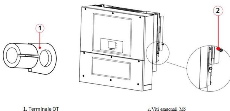
Figura 18 - Collegamento del terminale di terra
