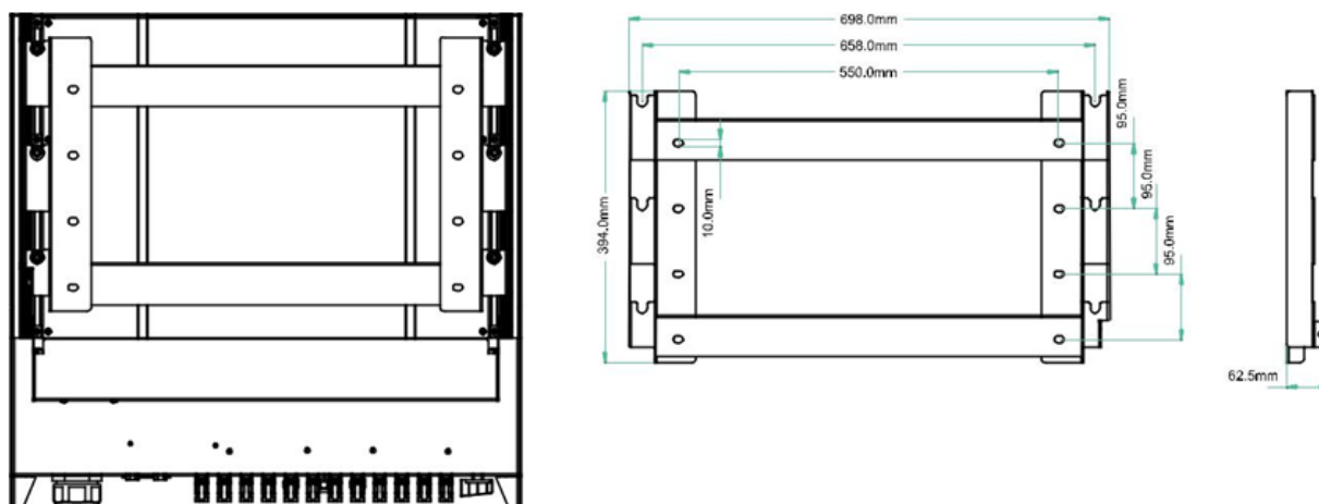
Figura 5 - Vista frontale, laterale e posteriore dell'inverter e della staffa
