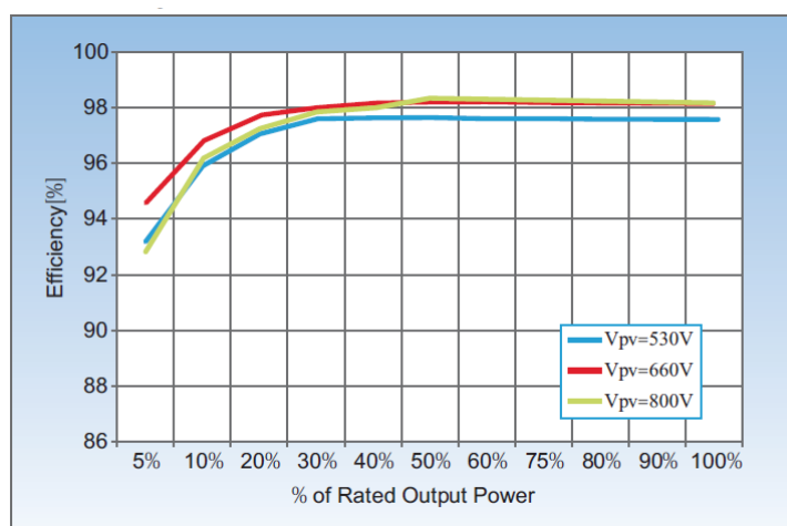
Figura 8 - Curva di efficienza per un inverter Azzurro ZCS della famiglia 3PH 50000TL-60000TL-V1
