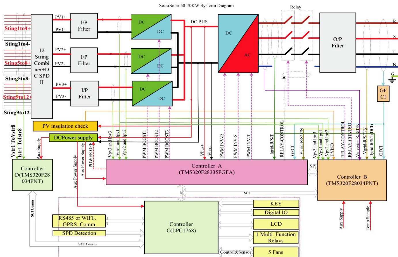
Figura 7 - Schema di funzionamento a blocchi degli inverter della serie 3PH 50000TL-60000TL-V1
