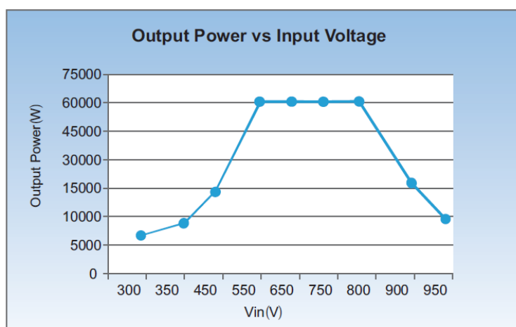
Figura 9 - Curva di derating della tensione in ingresso per un inverter Azzurro ZCS della famiglia 3PH 50000TL-60000TL-V1
